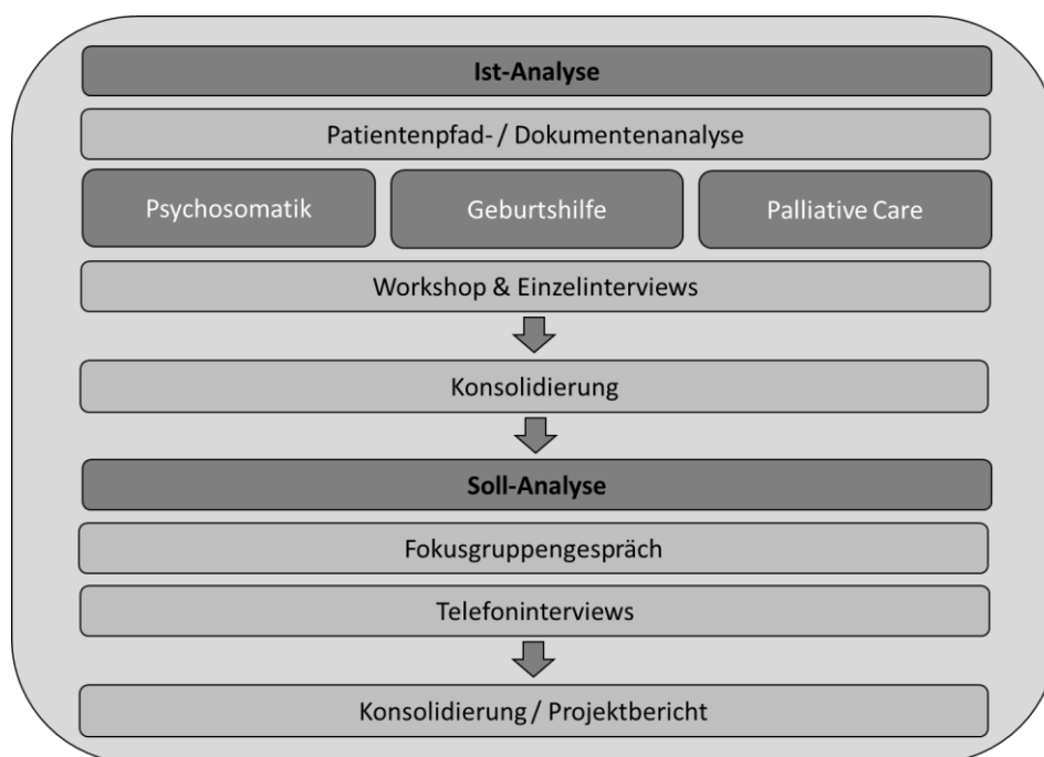
Abbildung 2 Sequentielle Projektstruktur.
