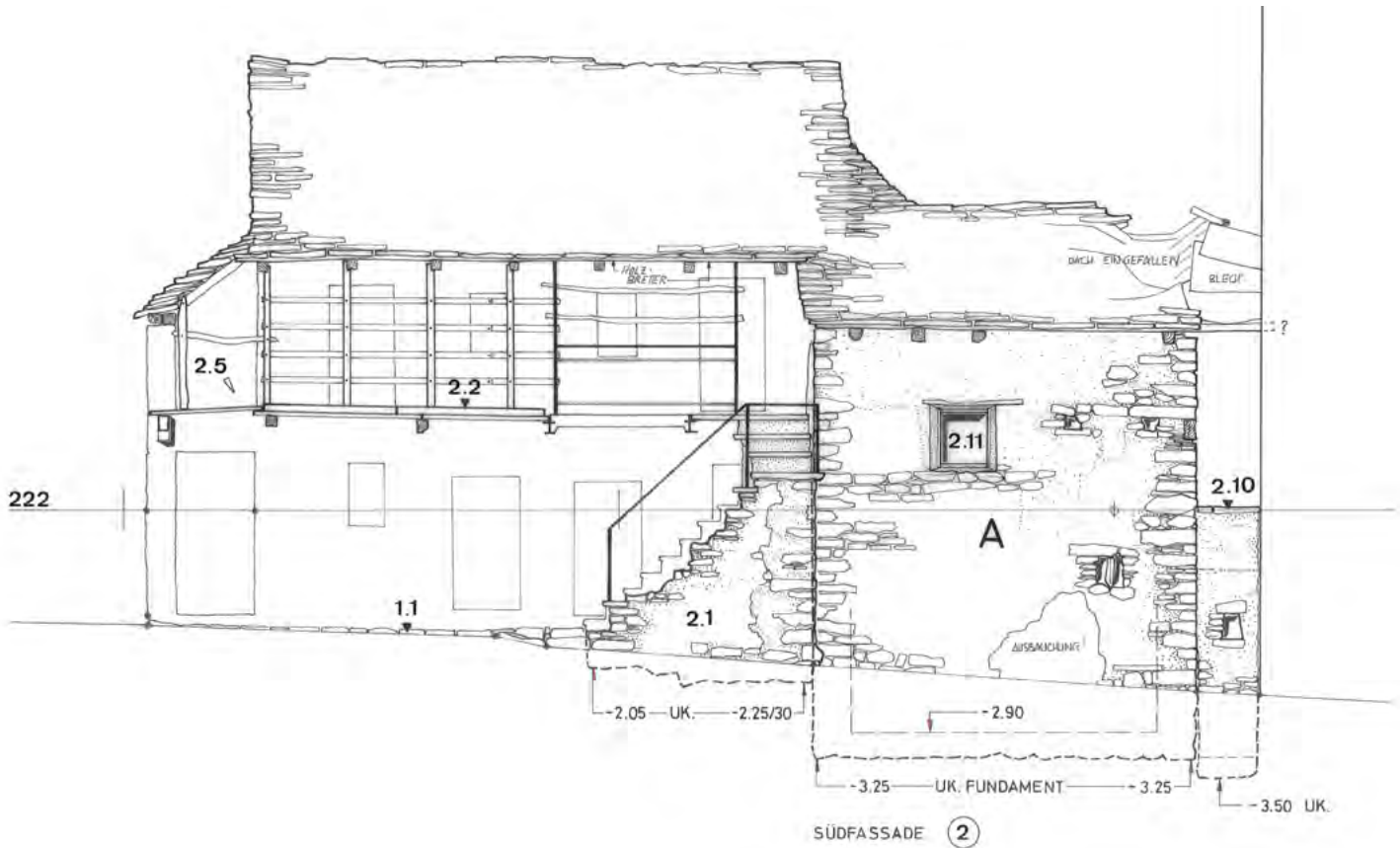
20 Cugnasco, Wohnhauskomplex: Aufnahmeplan, Südfassade Eckhaus, Plan 2.2. Aufnahme 2000.
