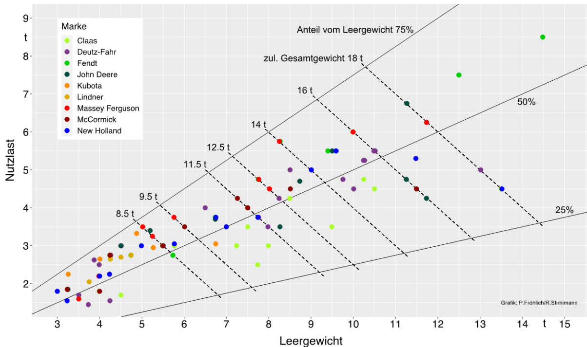
Bild 2: Nutzlast/Leergewicht-Verhältnisse von Traktorbaureihen ausgewählter Hersteller (© HAFL)
