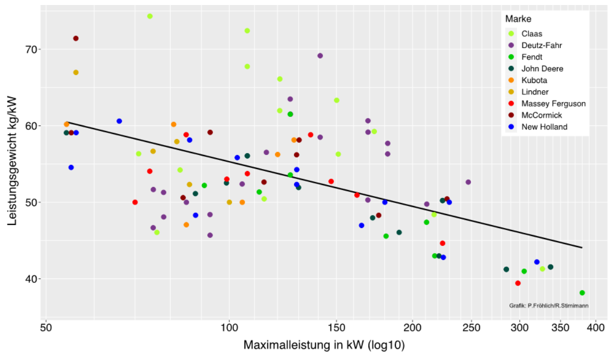
Bild 3: Leistungsgewichte von Topmodellen ausgewählter Hersteller (Quelle: HAFL)
