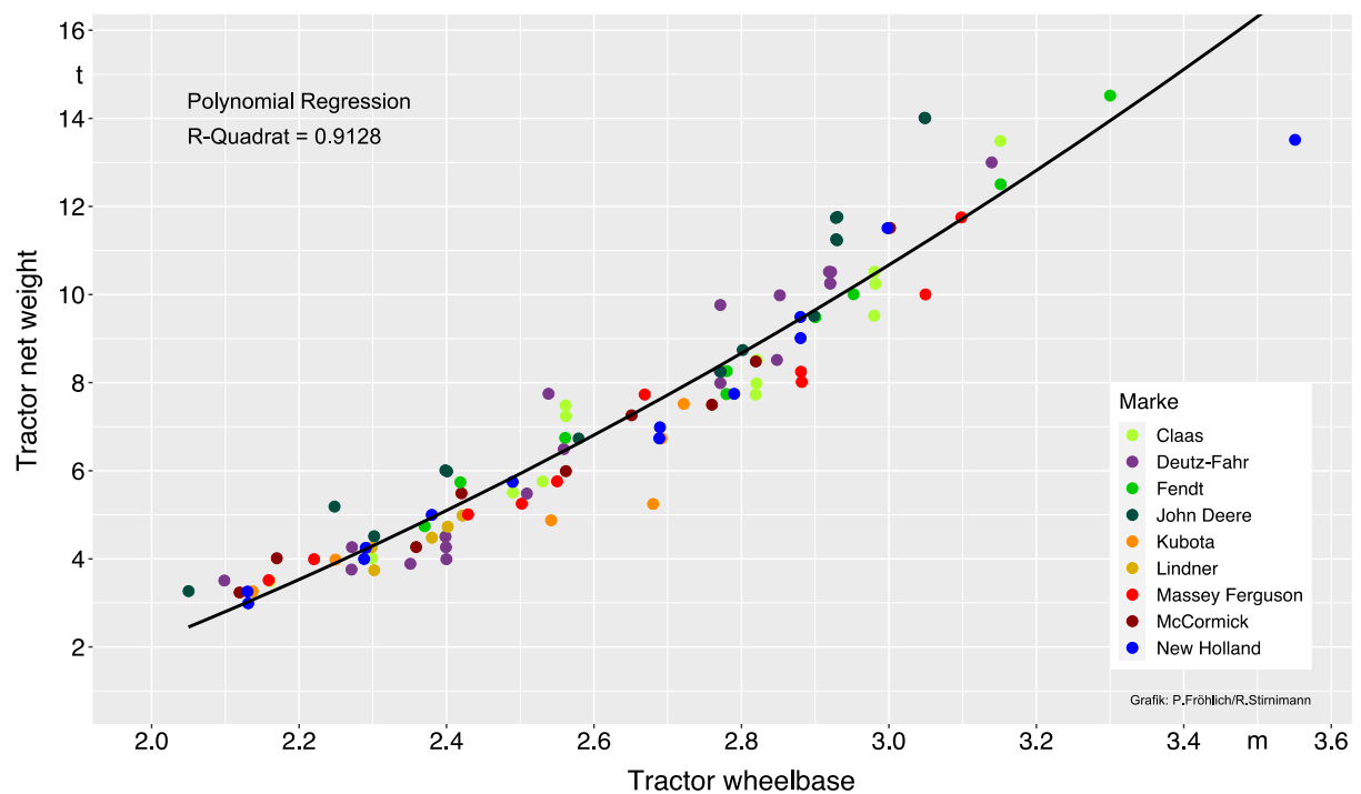
Bild 4: Leergewichte in Abhängigkeit der Radstände von aktuellen Traktorbaureihen (Quelle: HAFL)
