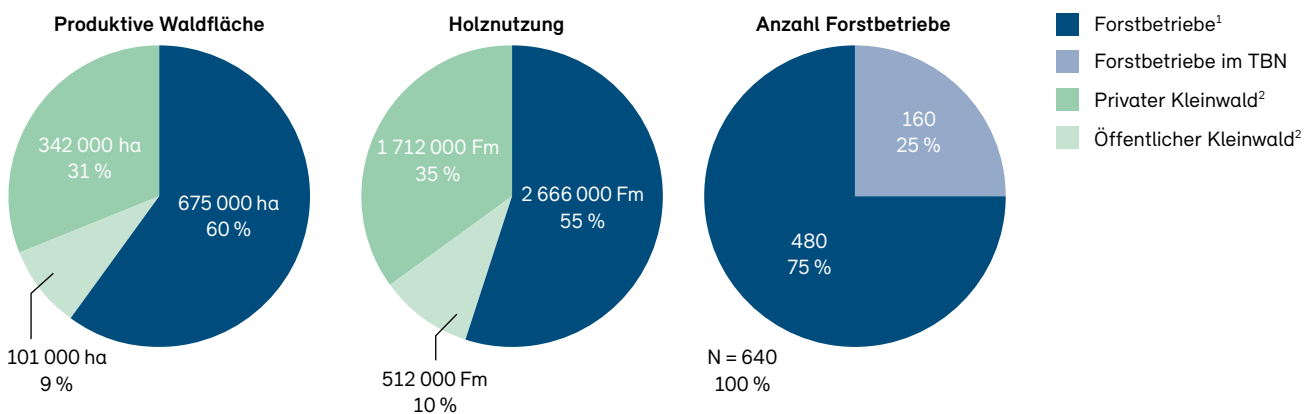
Grafik 10.1: Bewirtschaftungseinheiten 2023
