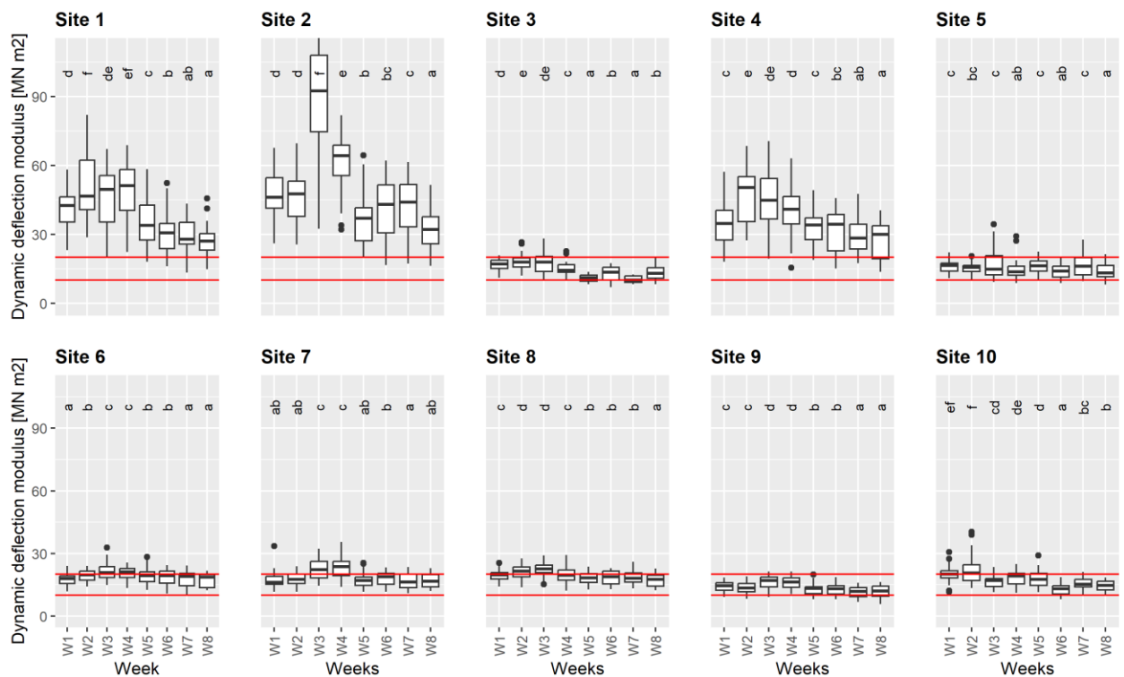
Fig. 2 : Résultat des modules de déformation dynamique Evd pendant 8 semaines sur 10 sols équestres, qui reflètent la dureté des sols. Les lignes rouges horizontales indiquent la plage de valeurs cibles pour la dureté des sols, entre 10-20 MN/m 2 .
