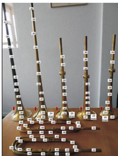
ABILDUNG 4 Fünf Schallstücke der Firma Egger, Basel. Ausgangsblechdicken: 0,45 mm für Nr. 1, 0,40 mm für die Nr. 2–5. 2 Steckbögen aus 0,50 mm-Blech
