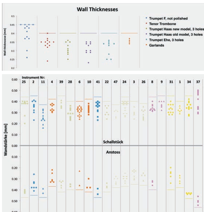
ABILDUNG 5 (oben) Gemessene Wandstärken an Egger-Schallstücken und -Kranzen (vgl. Abbildung 4) in tabellarischer Form
